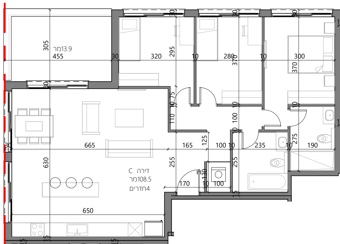
קומה טיפוסית - דירה C 1 : 100
